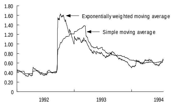
VaR estimate
